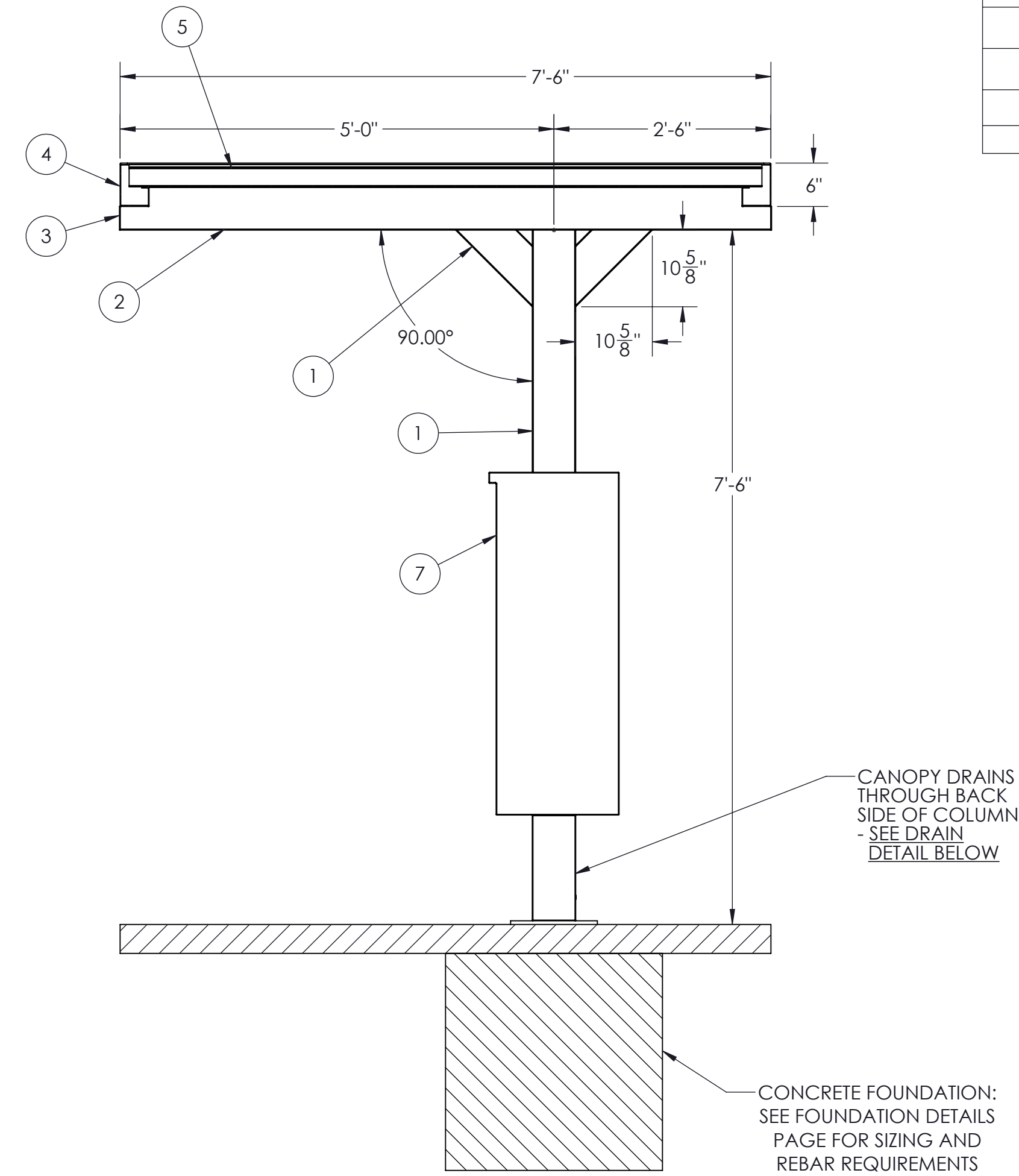
SECTION A-A SCALE 1:16
